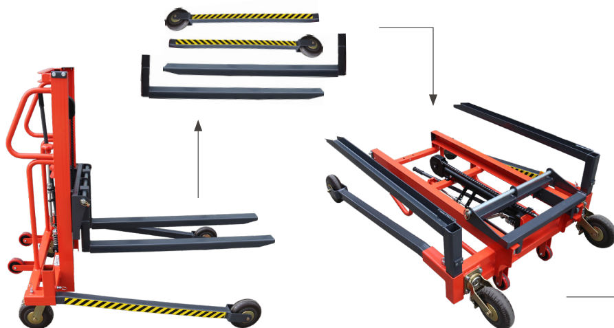
Fourches et longerons amovibles
