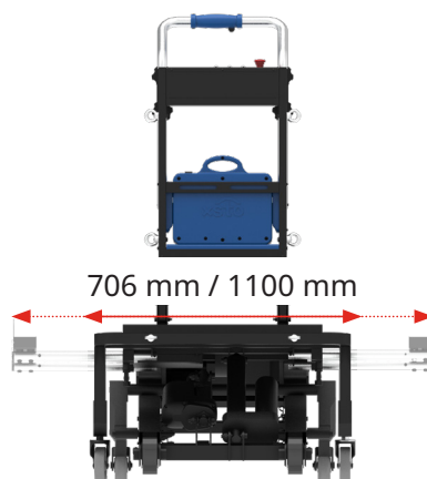
Plaque de chargement réglable
